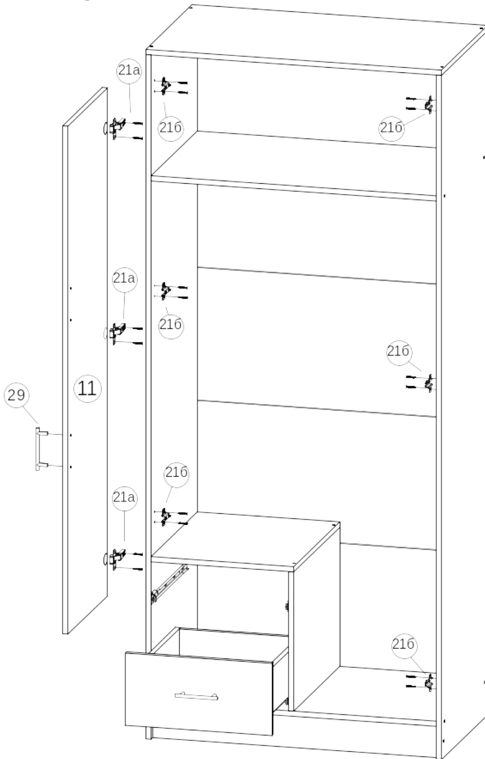
Рис.8 - Монтаж крестовины петли 21 на боковину
