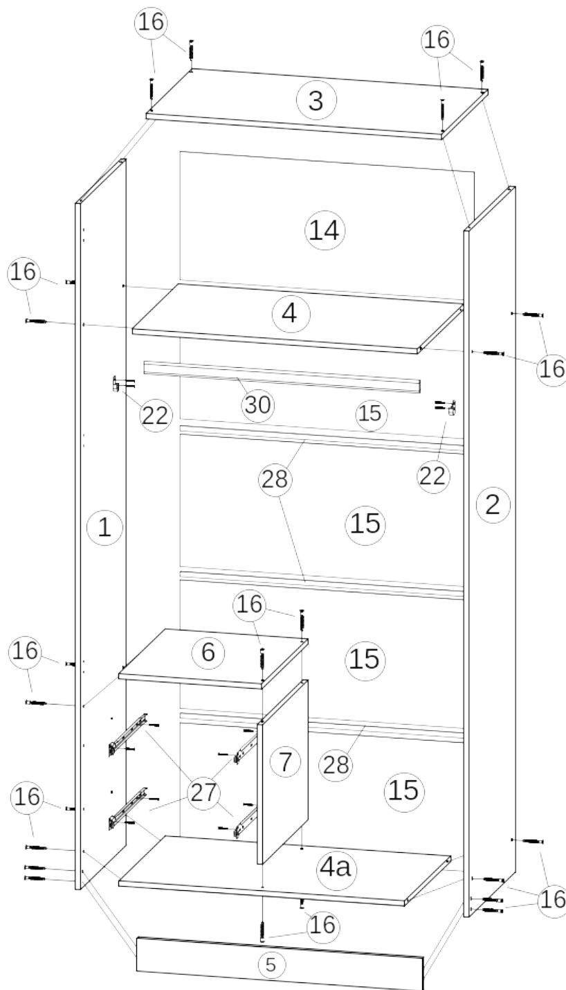
Рис.2 - Установка евровинта 16
